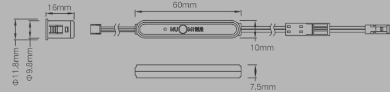
BẢN VẼ LẮP ĐẶT
